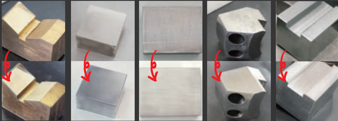
↑真鍮バリ取り ↑アルミの面取り ↑カッター目消し ↑超硬削り ↑キー溝のカッター目消し
